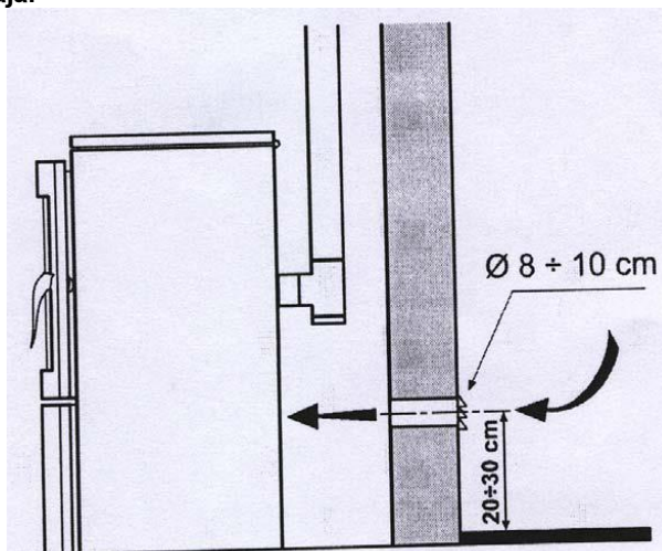
Slika 8. MINIMALNA RASTOJANJA ZA POSTAVLJANJE VENTILACIONE REŠETKE:
